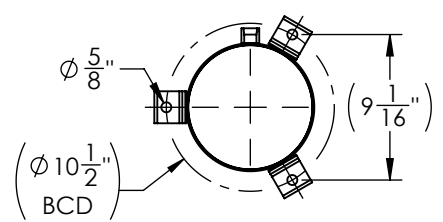
SECTION A-A SCALE 1 : 12
