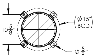
SECTION A-A SCALE 1 : 16
