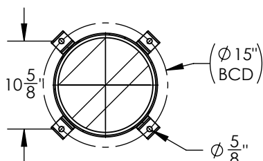
SECTION A-A SCALE 1 : 16
